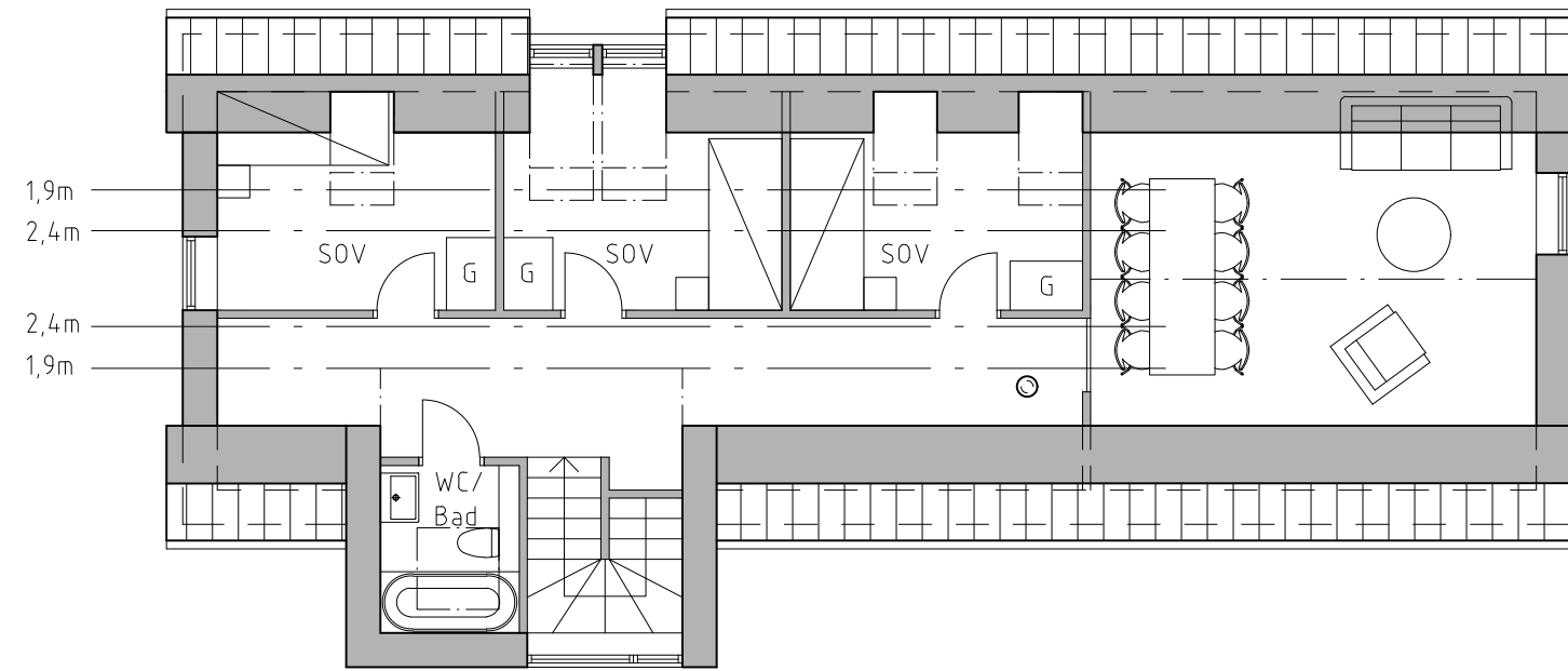
PLAN OVANVÅNING BOAREA: 48 KVM
