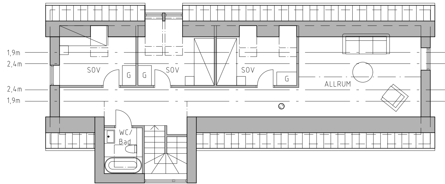
PLAN OVANVÅNING BOAREA: 67 KVM
