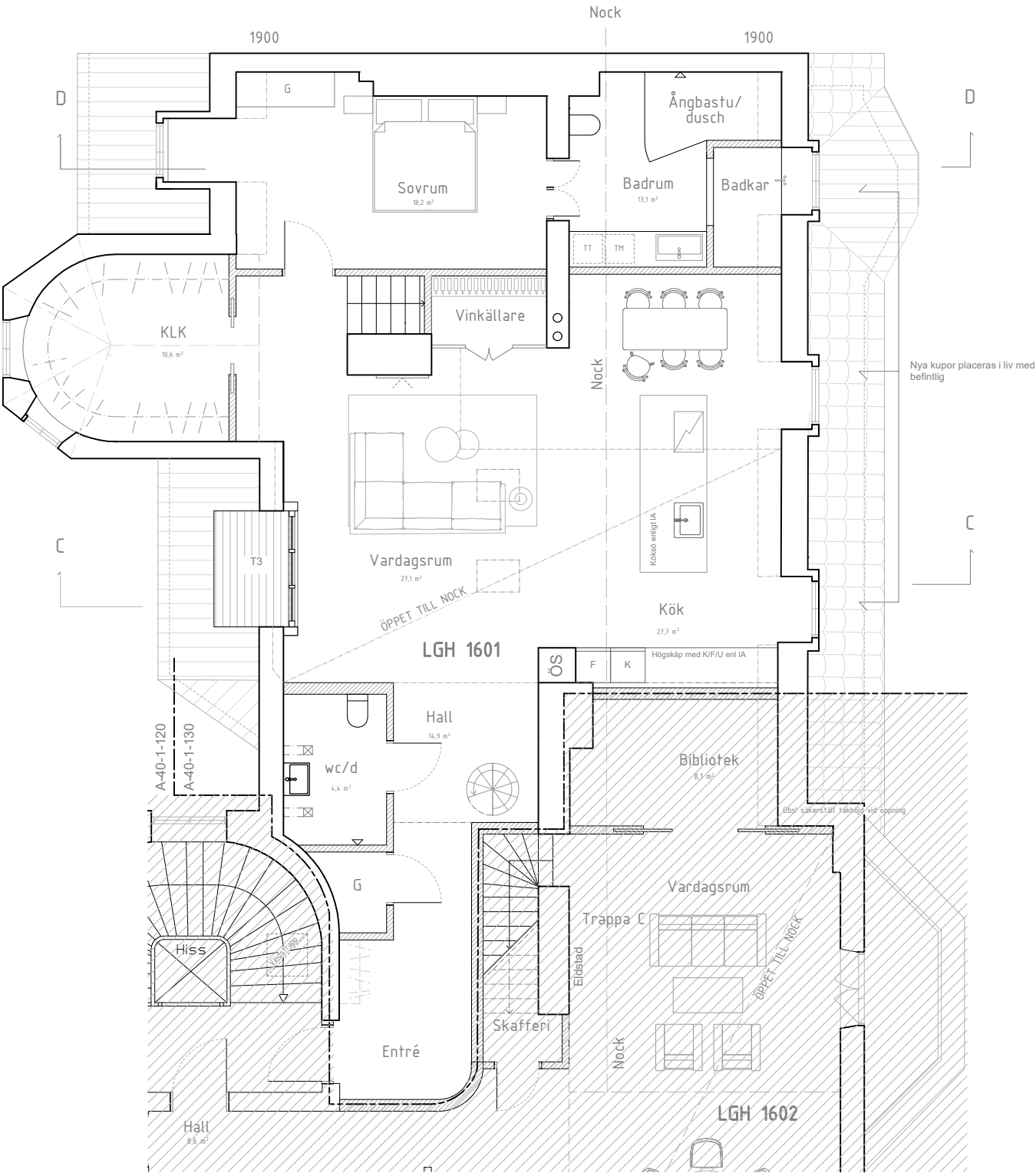
VINDSPLAN
