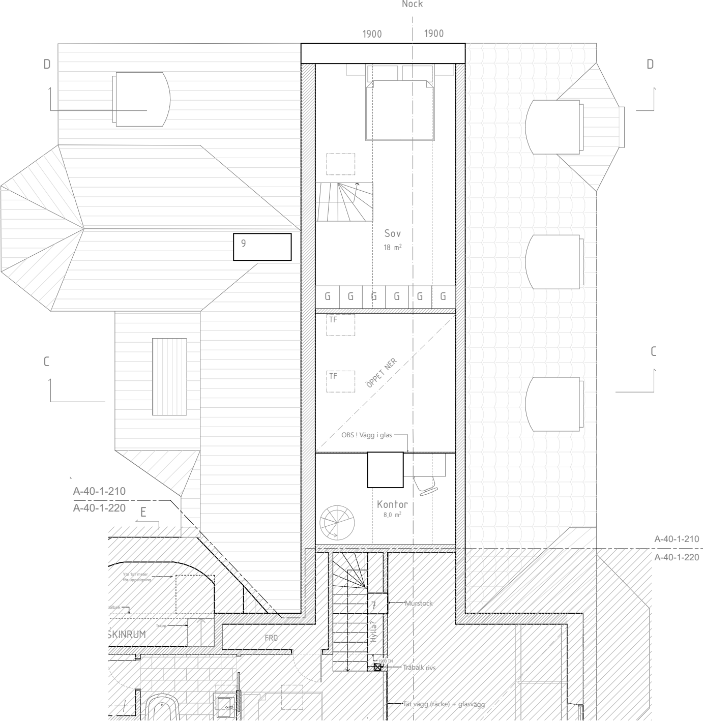
LOFTPLAN
