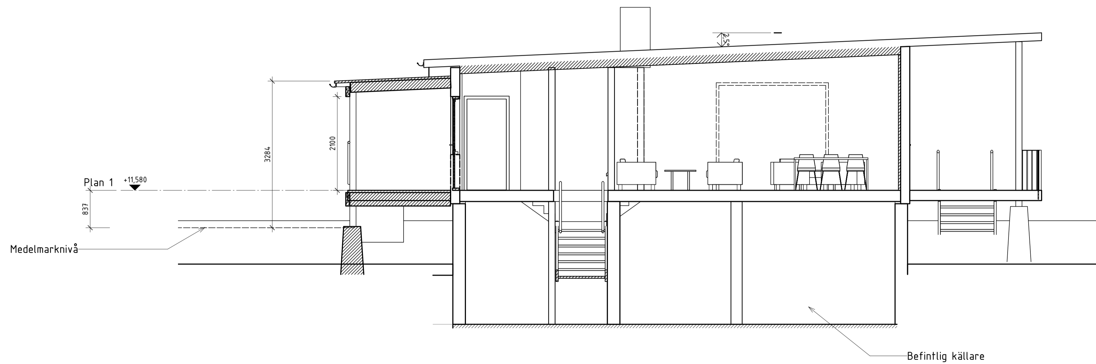
Sektion A-A
